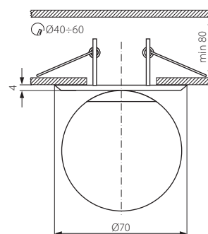
IGLO CTX-30+G-C/M
