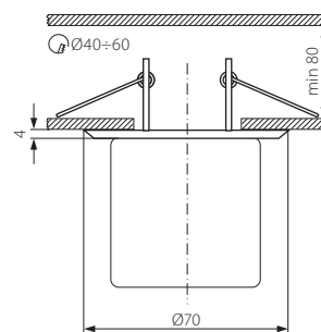
IGLO CTX-30+SQ-C/M
